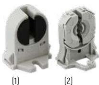
SUPORTE PARA LÂMPADA TUBULAR
